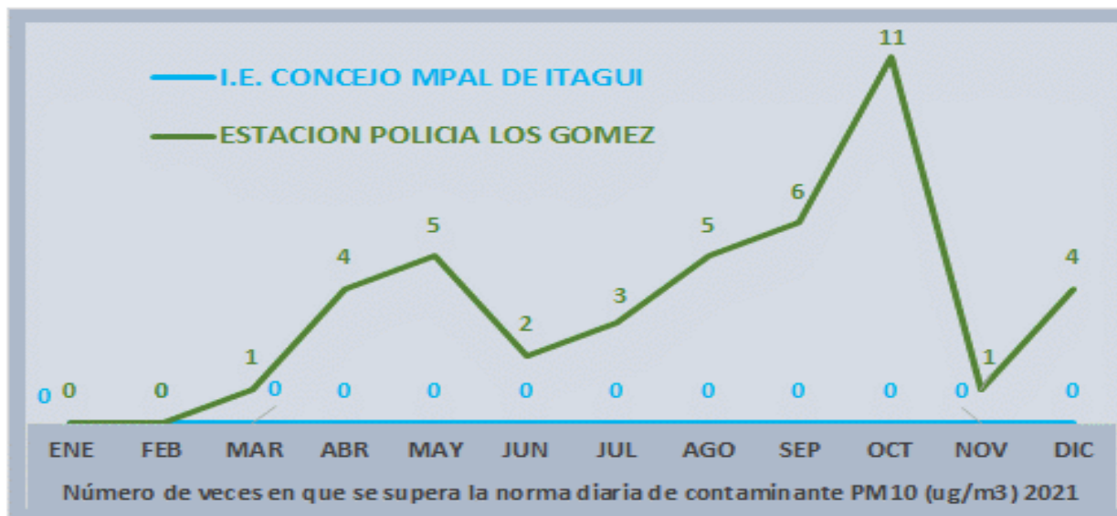
Gráfica 102. Número de veces en que se superó la norma diaria de contaminante PM10 (ug/m 3 ) 2021
