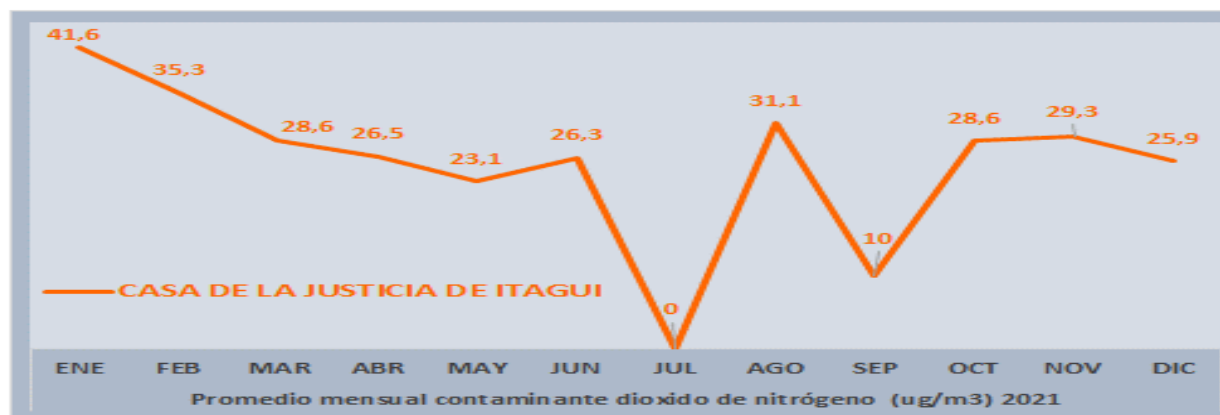
Gráfica 106. Promedio mensual de calidad del aire contaminante dióxido de nitrógeno ( \mu\text{g}/\text{m}^3 ), 2020.
